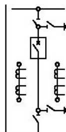
3BB-1000 3BB-600 3BB-400 Шинный ввод, секционный выключатель
