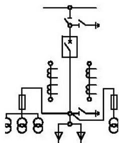
6.7BB-1000 6.7BB-600 6.7BB-400 Ввод, отходящая линия
