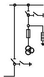
12.1-1000TH 12.1-600TH 12.1-400TH Трансформ. напряжения с боковым переходом
