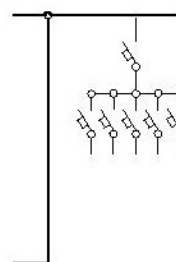
28.1А 28.4А Панель собственных нужд (28.1-задний, 28.4 - боковой переход)
