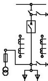
6.2BB-1000 6.2BB-600 6.2BB-400 Ввод, отходящая линия
