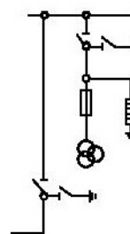
12.1-1000TH 12.1-600TH 12.1-400TH Трансформ. напряжения с боковым переходом
