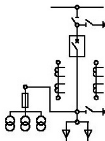
6.4BB-1000 6.4BB-600 6.4BB-400 Ввод, отходящая линия
