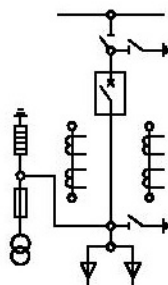
6.3BB-1000 6.3BB-600 6.3BB-400 Ввод, отходящая линия
