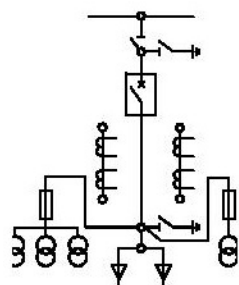
6.7BB-1000 6.7BB-600 6.7BB-400 Ввод, отходящая линия
