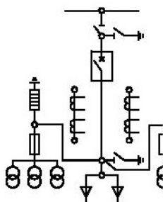
6.8BB-1000 6.8BB-600 6.8BB-400 Ввод, отходящая линия
